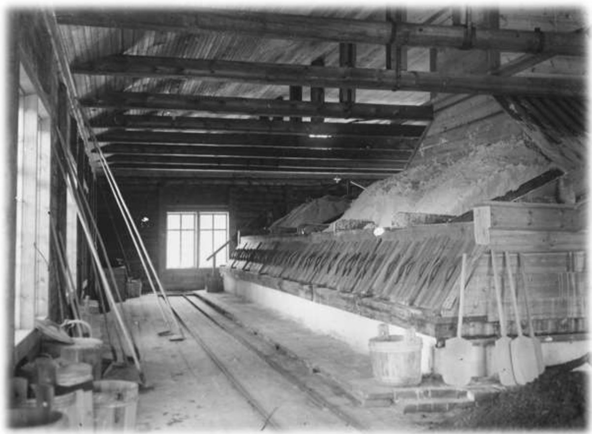
Технологическое устройство «белой» варницы
